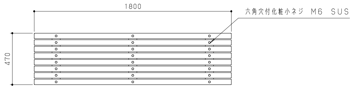
平面図 S = 1/20
